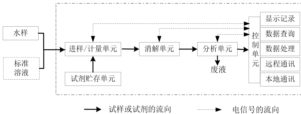
图 1 仪器的基本组成单元
